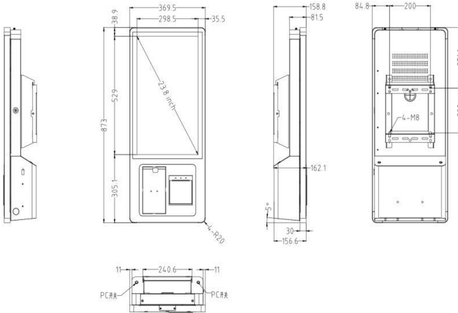
正视图
